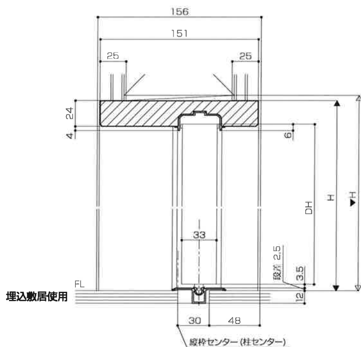
●縦断面図
