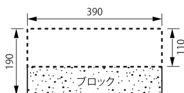
【図 1】開口部サイズ
