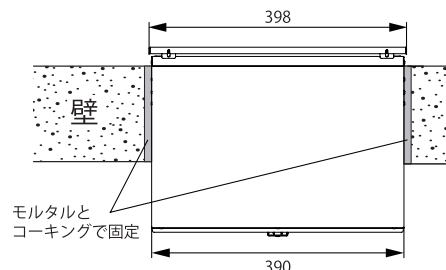
【図 2】施工時(上面図)
