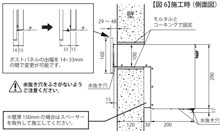
【図 6】施工時 (側面図)
