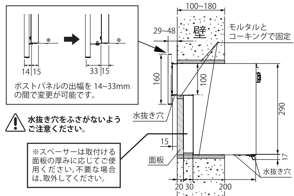
【図 4】ポストパネル取付・取外方法
