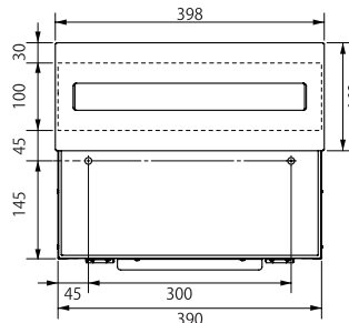
【図 2】オスト 15 タイプ 壁面接合部・ビス穴位置略図
