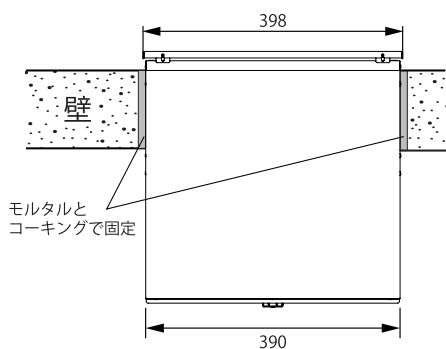
【図 5】施工時 (上面図)
