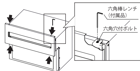
【図 4】ポストパネル取付・取外方法
